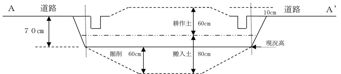
(改良断面図)
