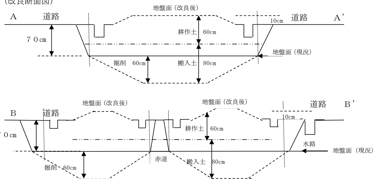
(改良断面図)
