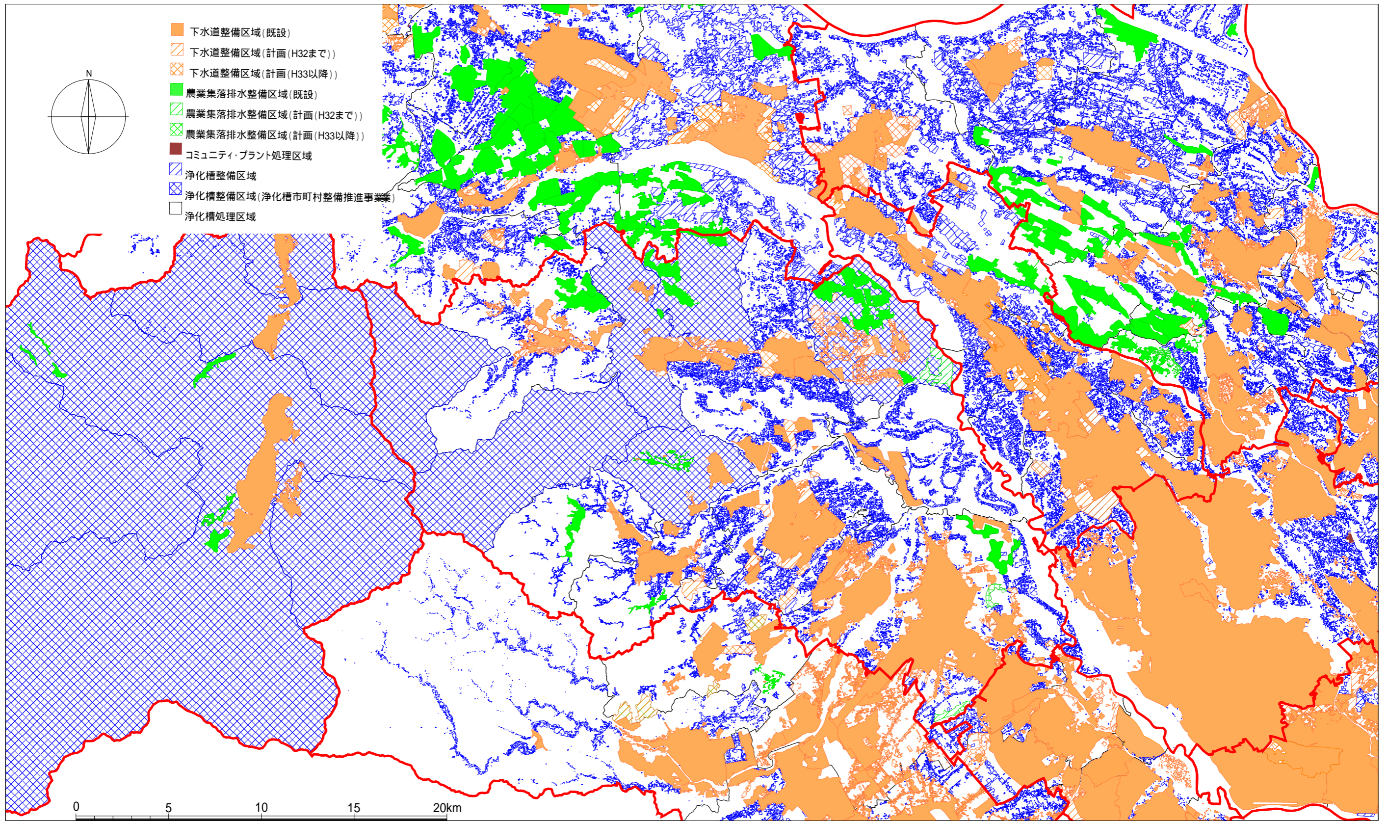
埼玉県生活排水処理施設整備構想図(川越比企地区) 1:200000
