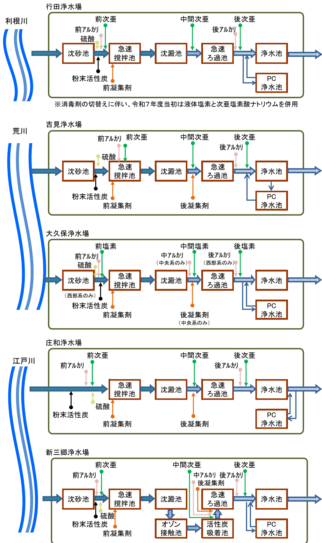
図1 浄水処理方法の概要
