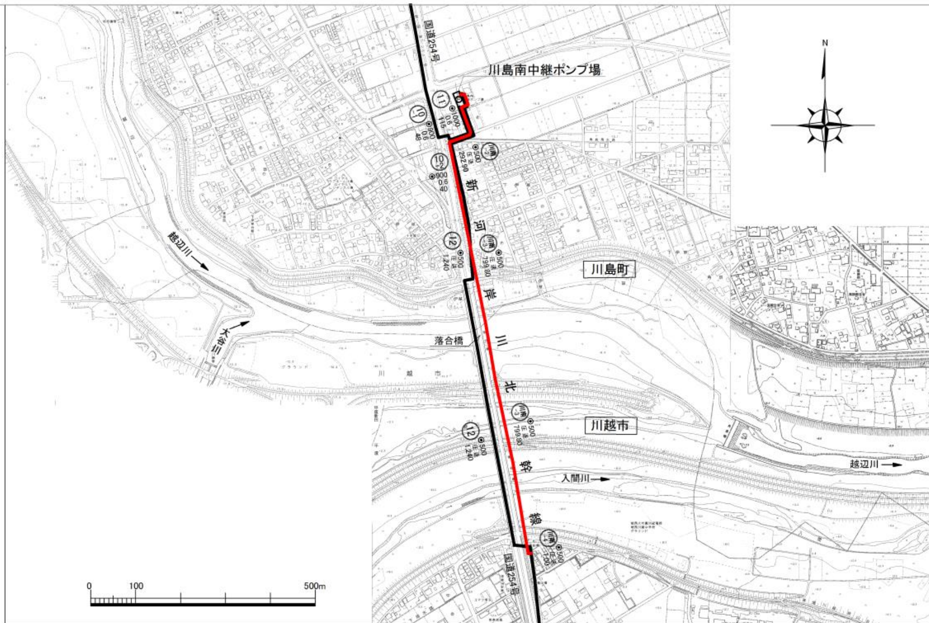
新河岸川北幹線(圧送管二条化)追加 ◎500 L=約1,090m
