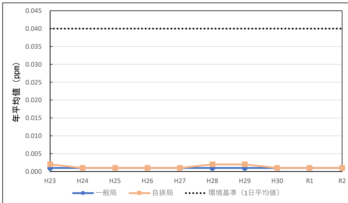
図 1 二酸化硫黄の年平均値の推移グラフ(10年継続測定局)
