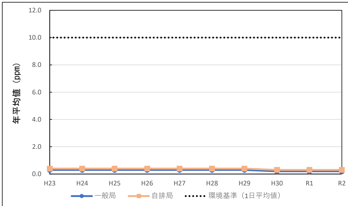
図3 一酸化炭素の年平均値の推移グラフ(10年継続測定局)
