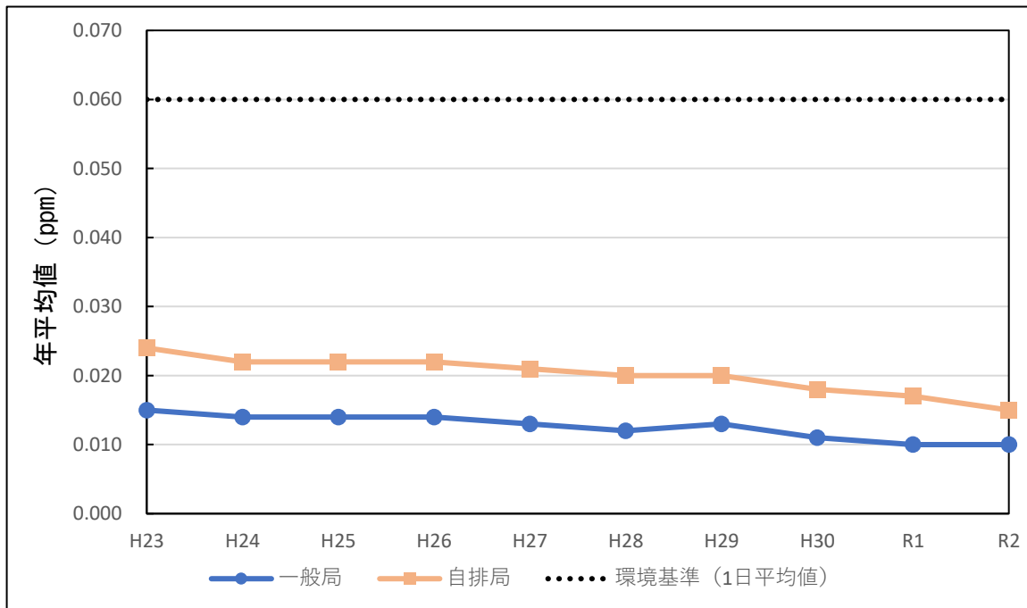
図2 二酸化窒素の年平均値の推移グラフ(10年継続測定局)
