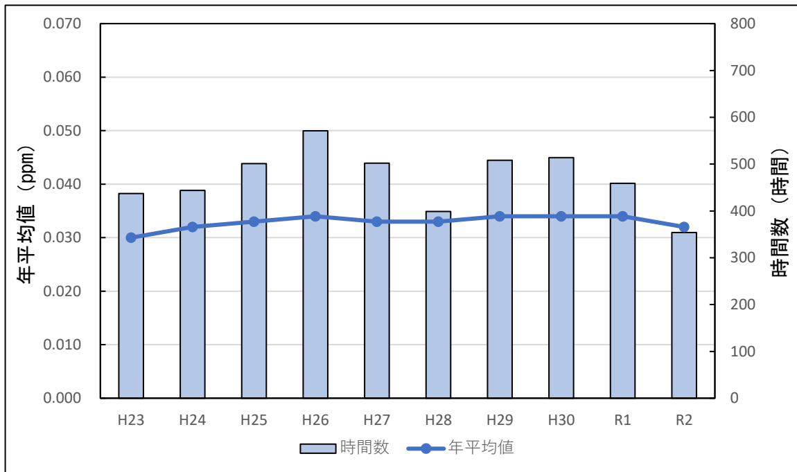
図4 光化学オキシダントの10年継続測定局における昼間の1時間値 (注) の年平均値及び昼間の1時間値が0.06ppmを超えた時間数の推移グラフ
