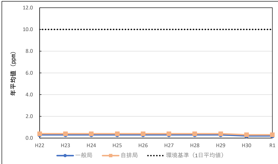
図3 一酸化炭素の年平均値の推移グラフ(10年継続測定局)
