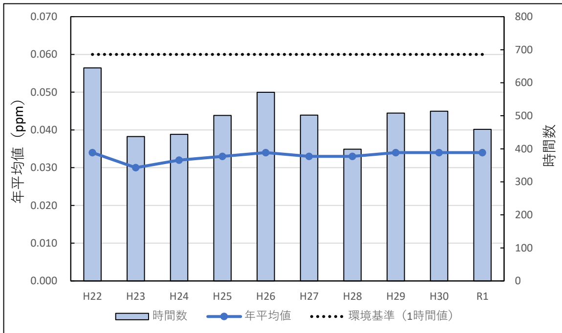
図4 光化学オキシダントの10年継続測定局における昼間の1時間値の年平均値及び昼間の1時間値が0.06ppmを超えた時間数の推移グラフ
