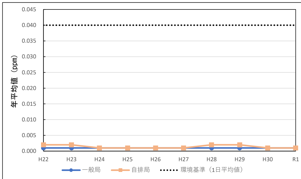
図1 二酸化硫黄の年平均値の推移グラフ(10年継続測定局)
