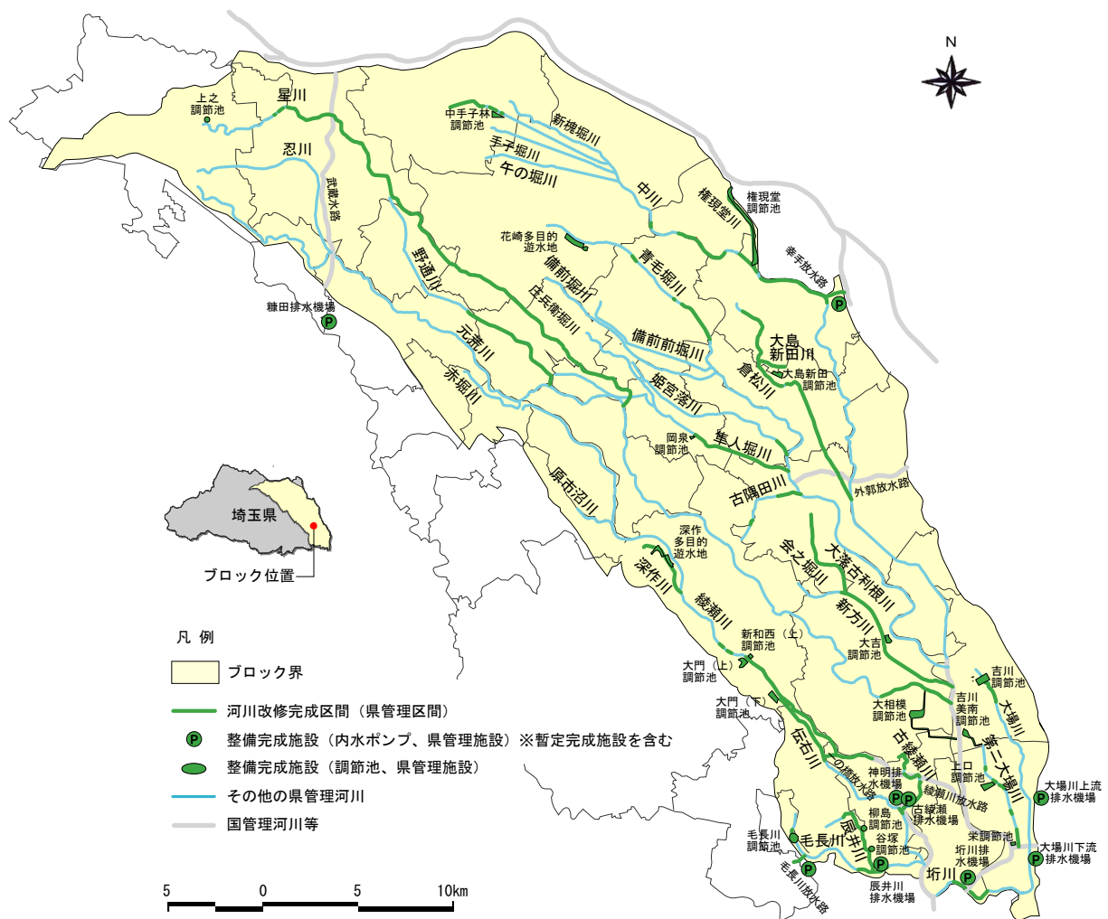
図1-7 なかがわ 中川・ あやせがわ 綾瀬川ブロックの河川整備状況(令和5年度末)
