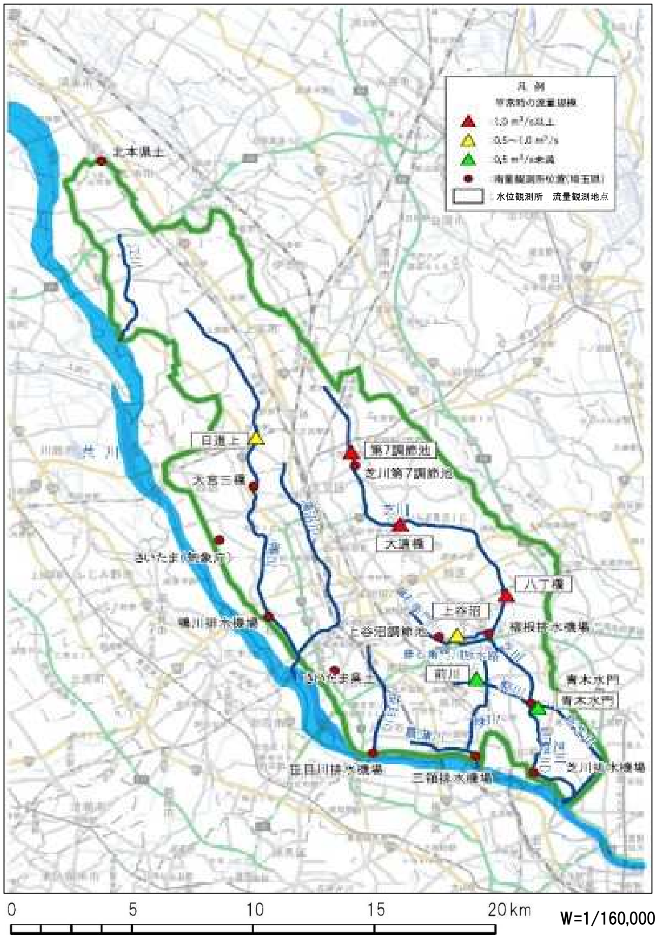
図 1.2.4 荒川左岸ブロック水位・流量観測所位置図
