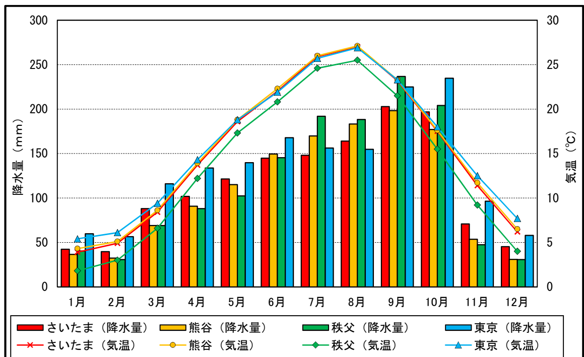
22 図 1.1.4 月別降水量と月別平均気温
