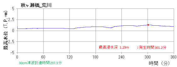
图 10.3.6-8(1) 代表地点波形 (水門閉鎖)
