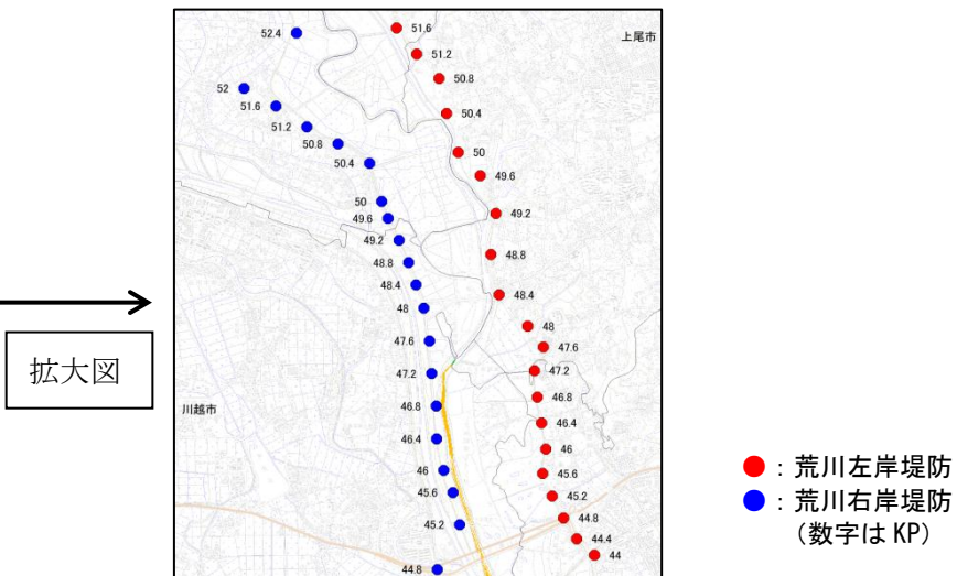
図 10.3.6-2 遡上結果図 (水門閉鎖)
