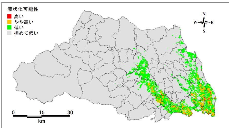
図 5.4-1(1) 液状化可能性分布図 (海溝型地震)
