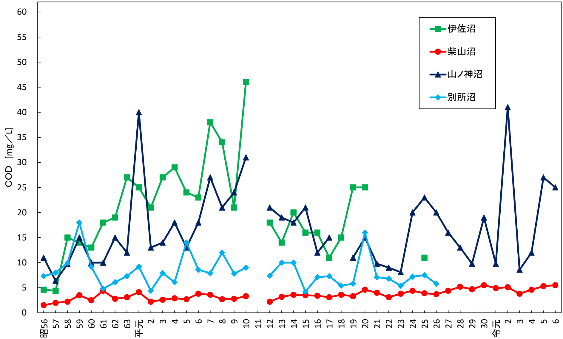
湖沼表層水のCOD経年変化（天然湖沼・冬季）
