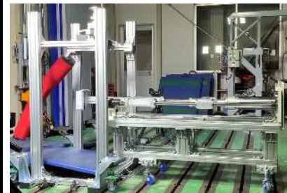
電動式水平射出装置を用いた 校正試験機を開発
