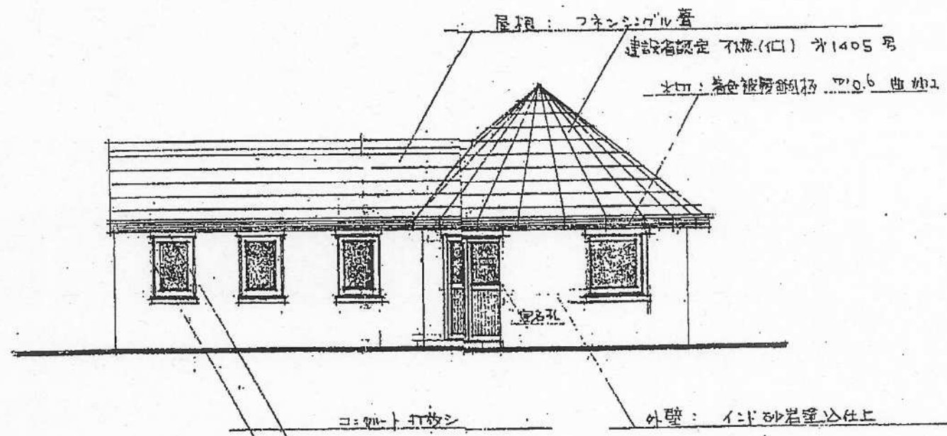
事務室 西立面図
