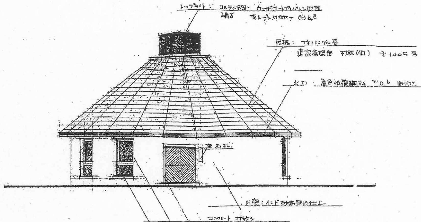
学習室 東立面図
