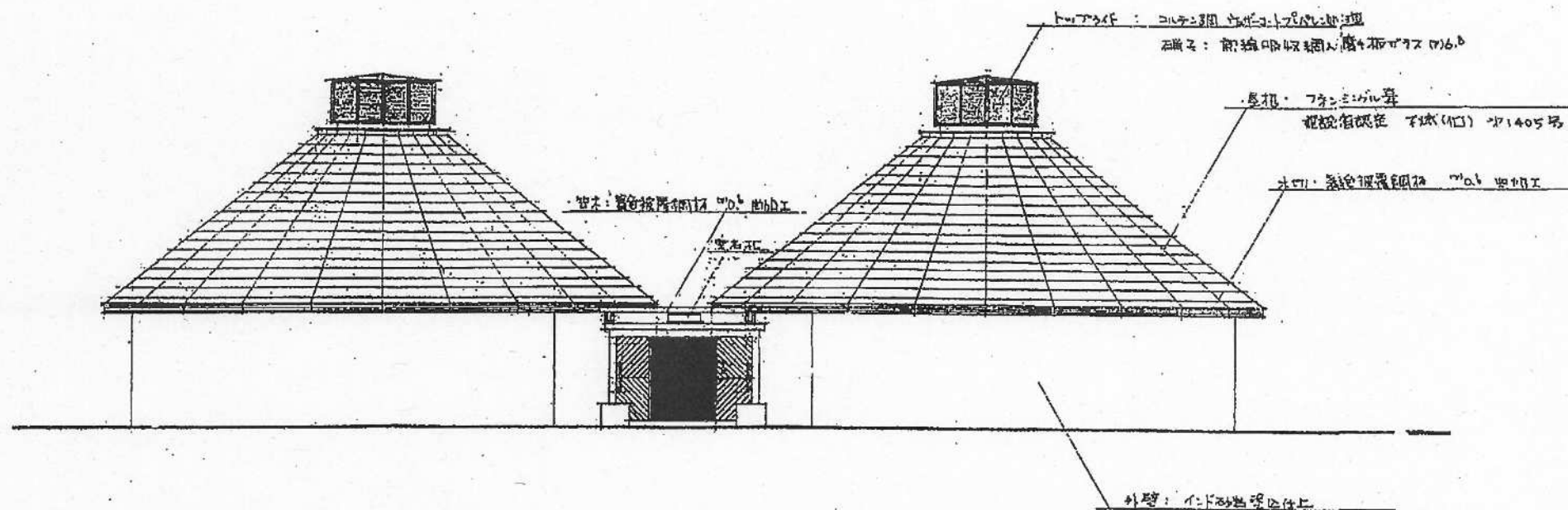
展示室 南立面図
