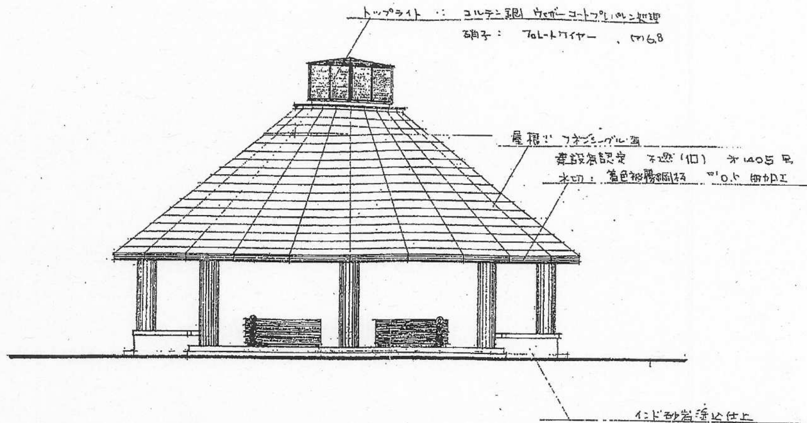
ホール 東立面図
