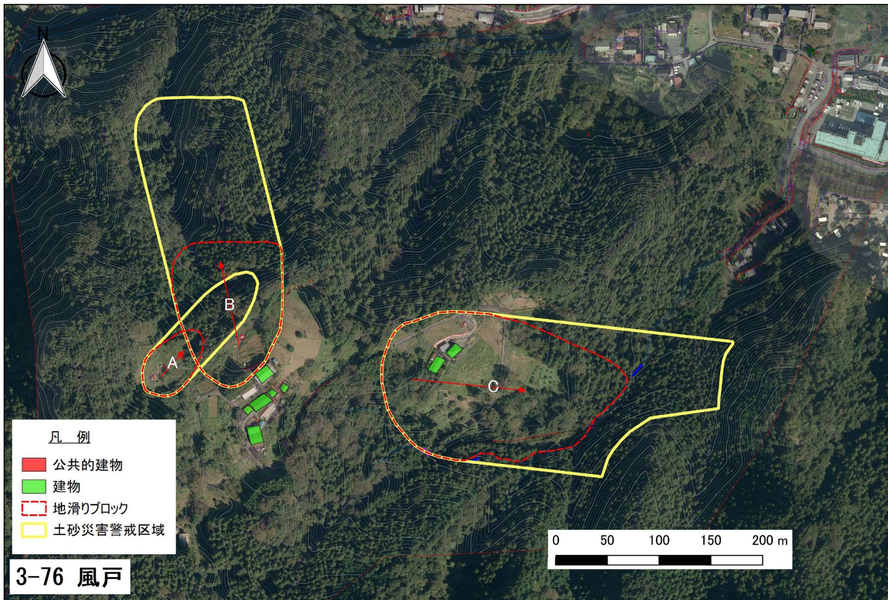
3-76 風戸 総括図
