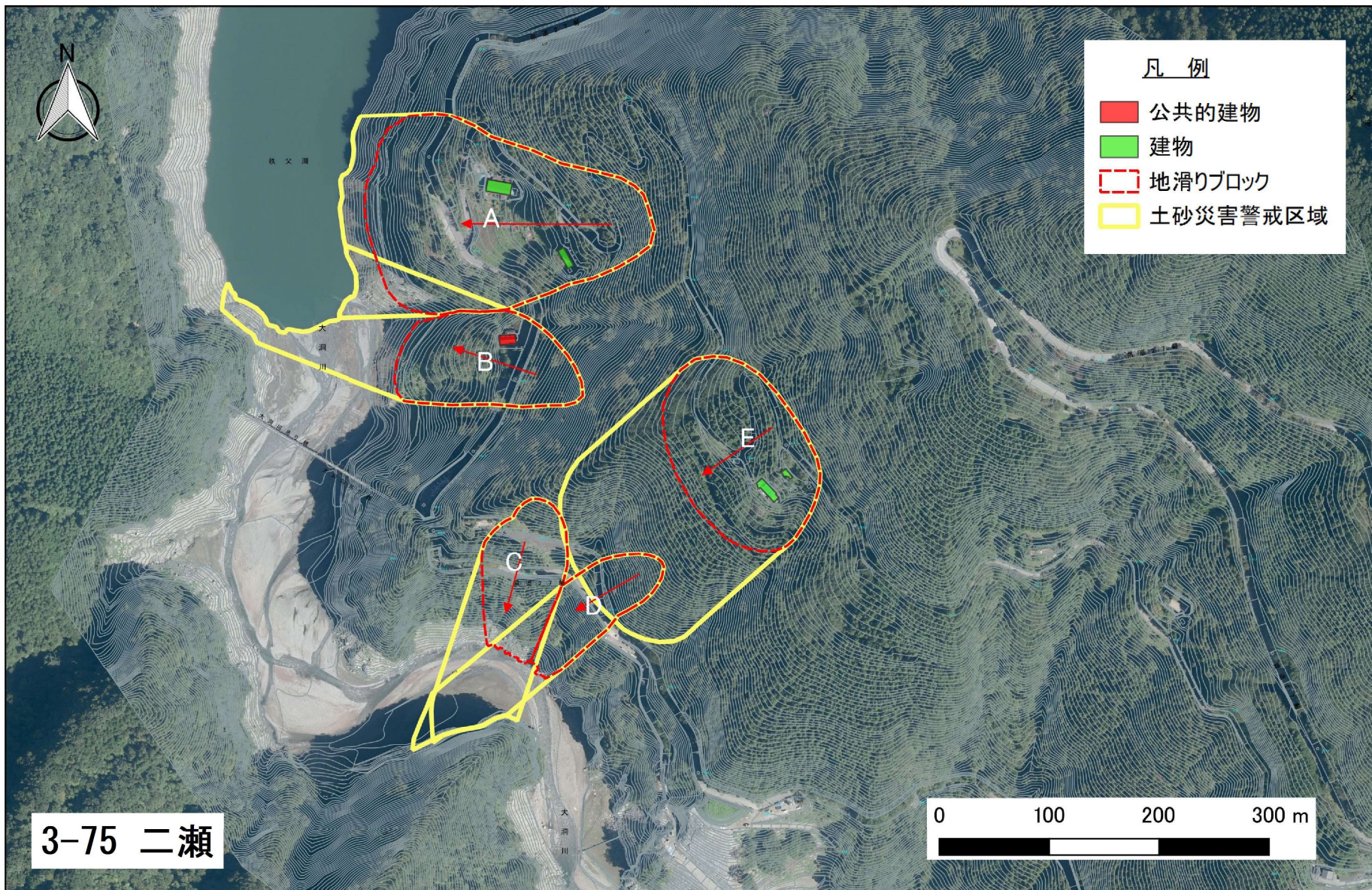
3-75 二瀬 総括図
