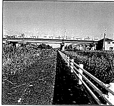
県管理貯水池側、約1kmにわたり防草シートを敷設
