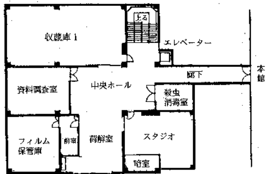
収蔵棟1階平面図
