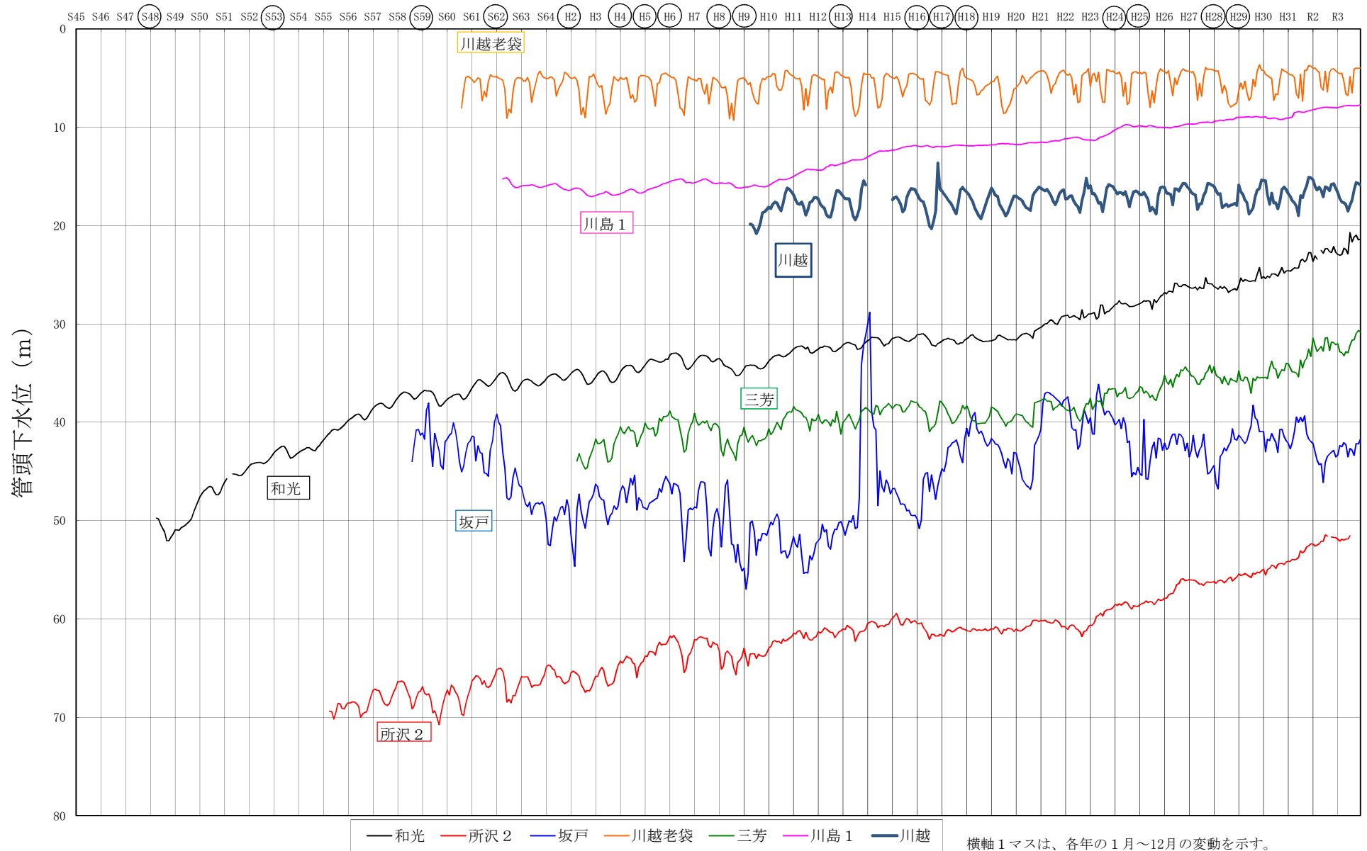
図 1-15 管頭下水位経年変化（西部・比企地域）（○印は渇水年）
