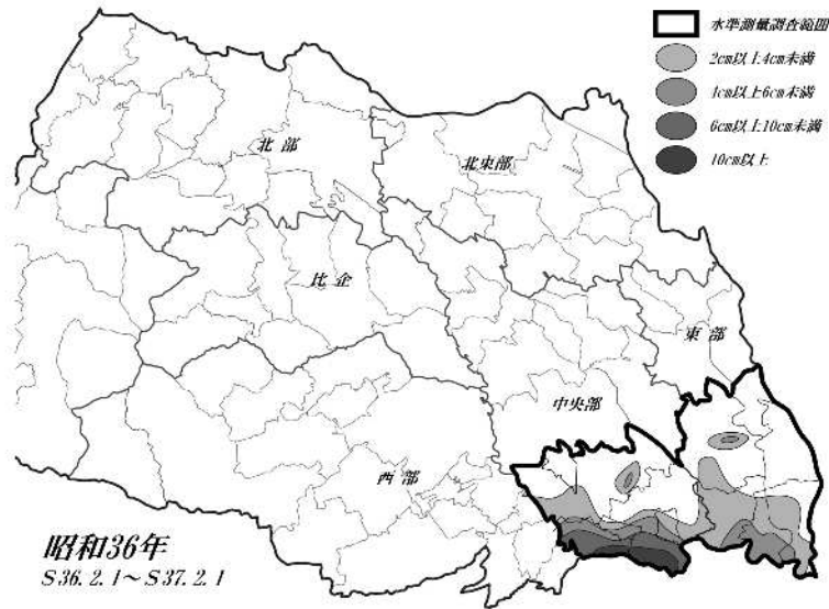
図1-11 地盤沈下地域の経年変化図
