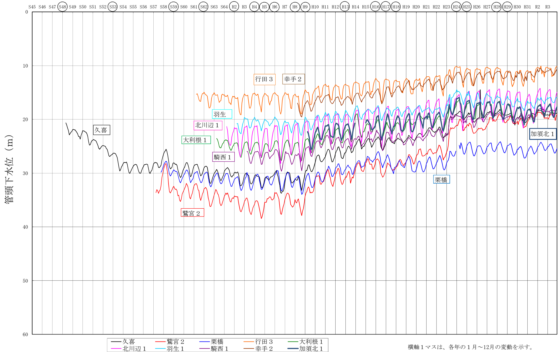
図 1-16 管頭下水位経年変化（北東部地域）（○印は渇水年）
