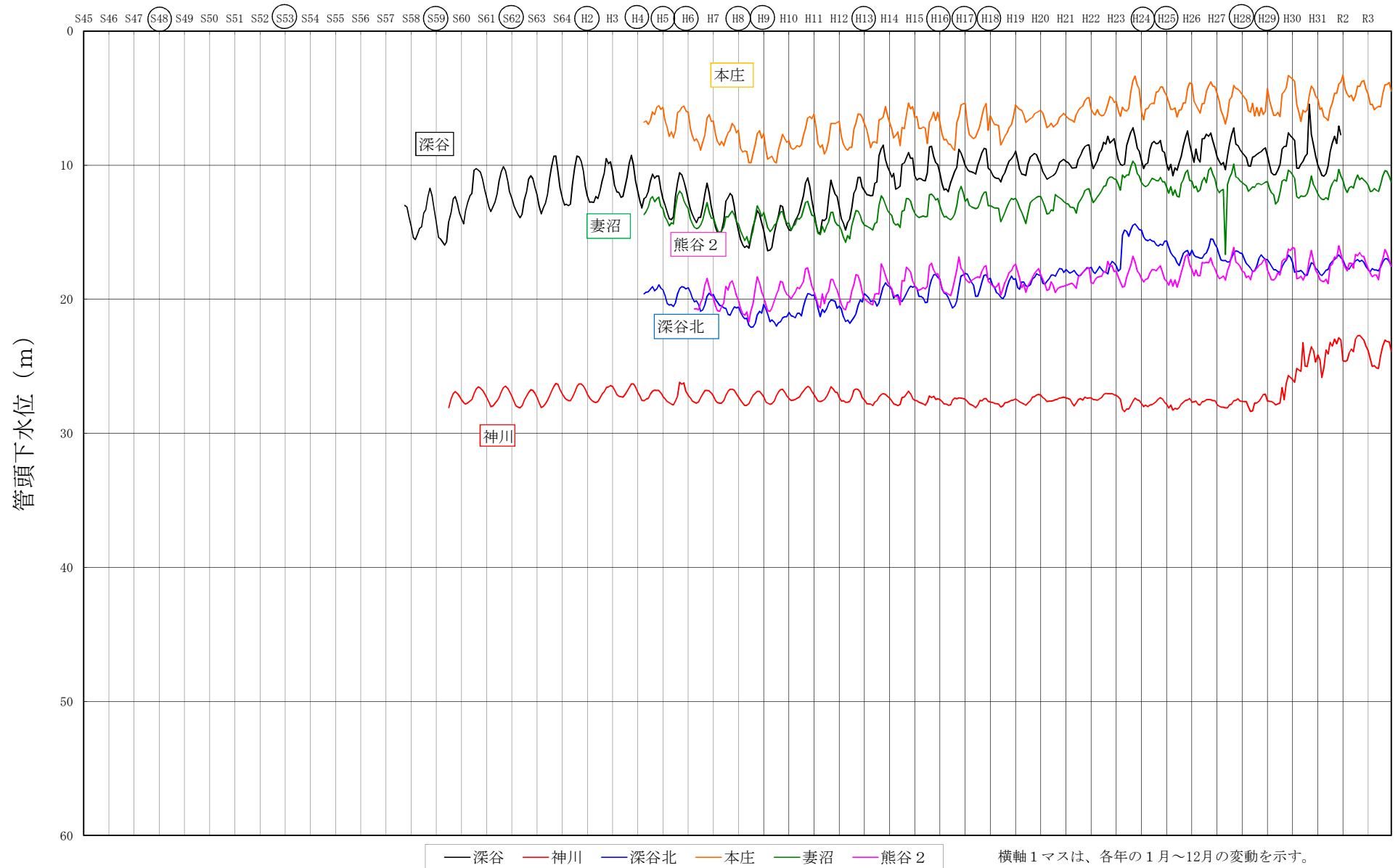
図 1-17 管頭下水位経年変化（北部地域）
