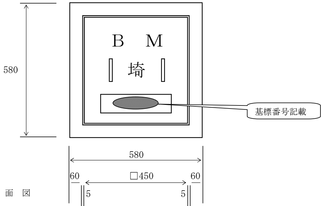
平面图
