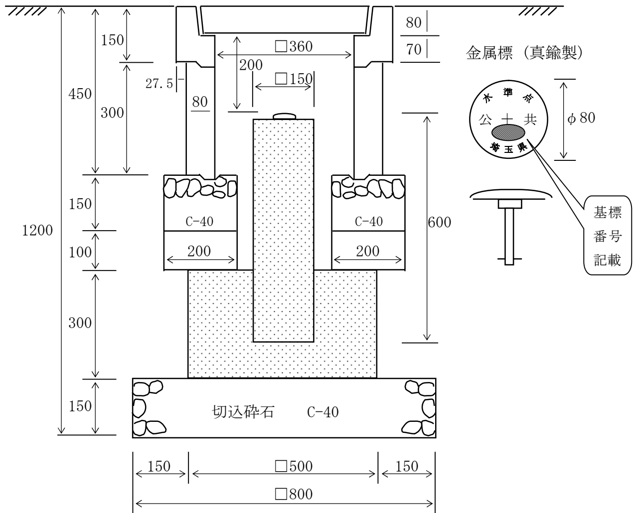
断面図
