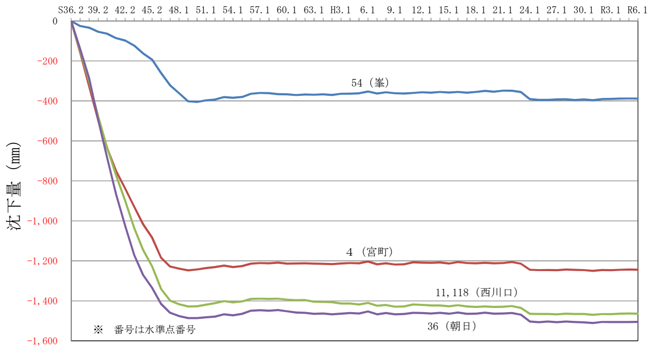
図 1－5 地盤沈下経年変化図（川口市） 測量基準日（年. 月）
