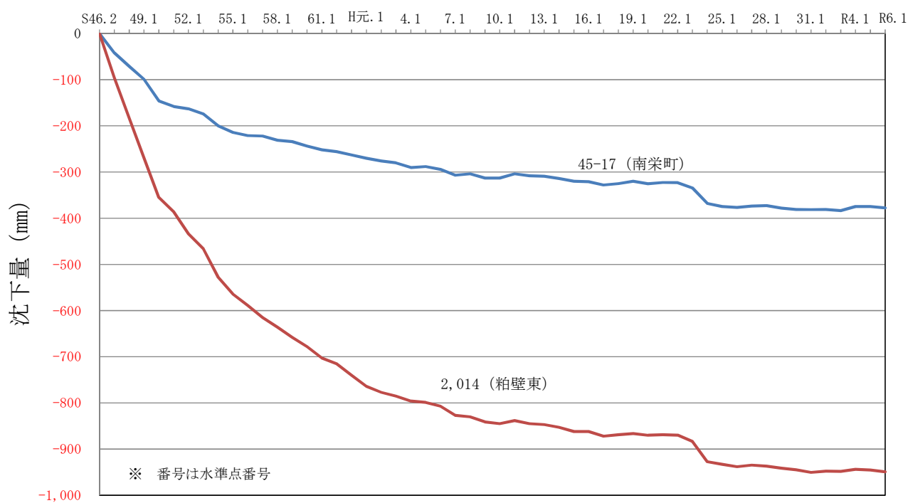
図 1 - 4 地盤沈下経年変化図（春日部市）
