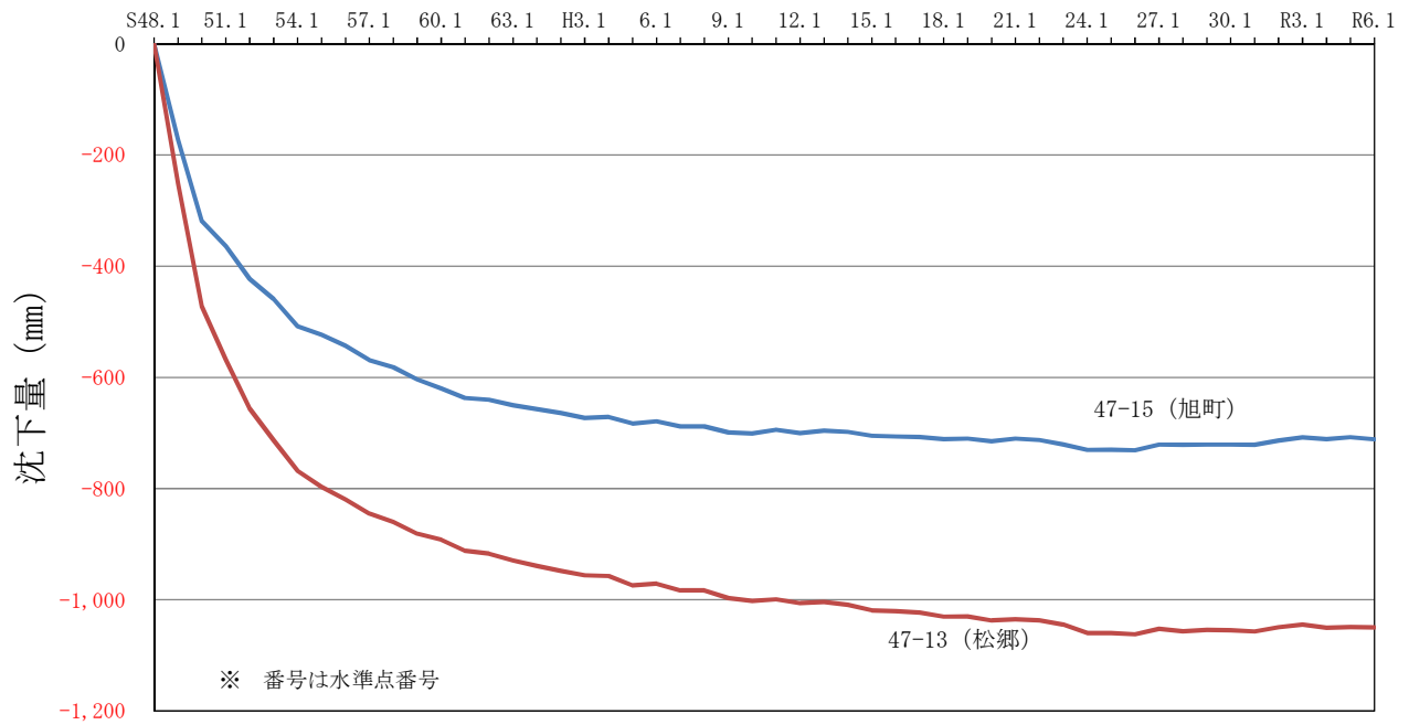
図 1 - 7 地盤沈下経年変化図（所沢市）
