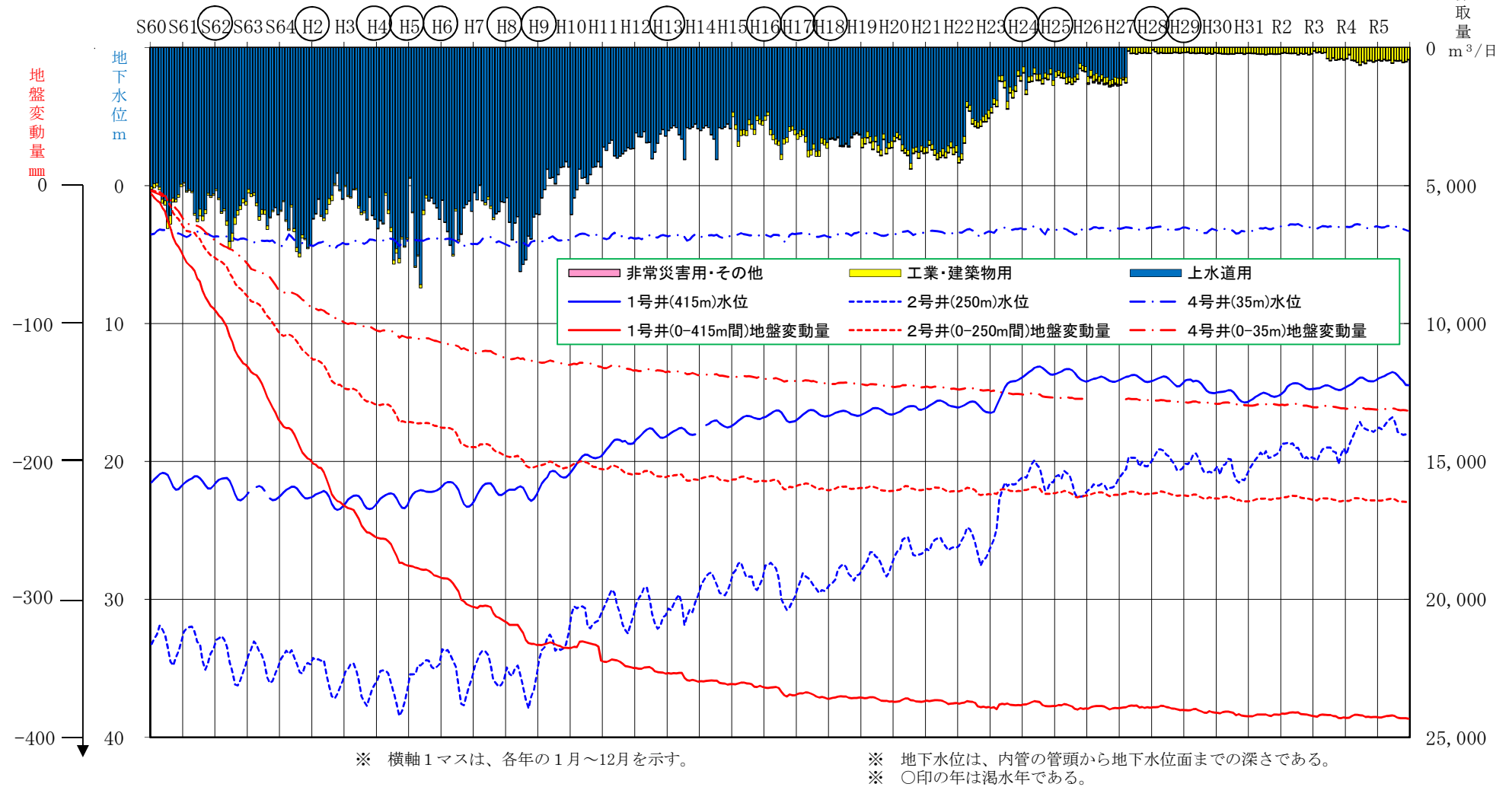
図 1 - 21 地下水採取量・地下水位・地盤沈下の相関図（久喜市（旧鷺宮町））（鷺宮観測所）
