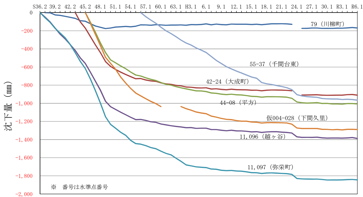
図 1 - 3 地盤沈下経年変化図（越谷市）
