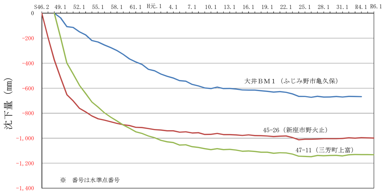
図 1 - 8 地盤沈下経年変化図（ふじみ野市、新座市、三芳町）
