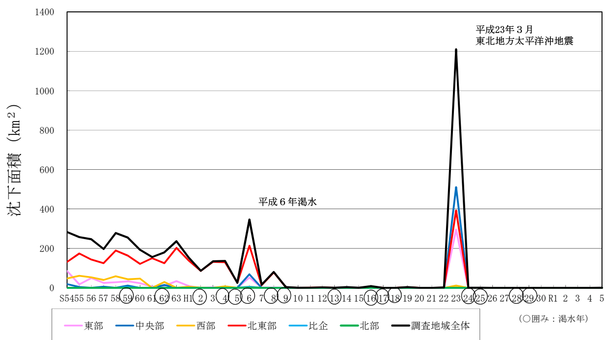
図 1－10 地域別沈下量面積（年 2 cm以上）の経年変化図
