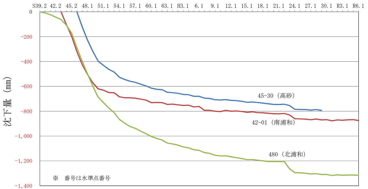
図 1－6 地盤沈下経年変化図（さいたま市） 測量基準日（年. 月）
