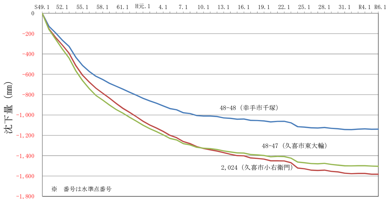
図 1－9 地盤沈下経年変化図（幸手市、久喜市）
