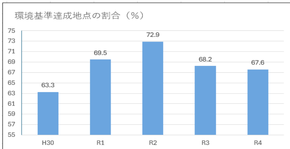
図2 過去の環境基準値以下の比率(点的評価)
