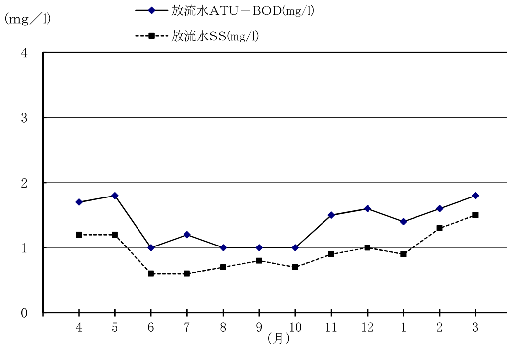
図6-8 令和5年度 放流水 BOD・SS
