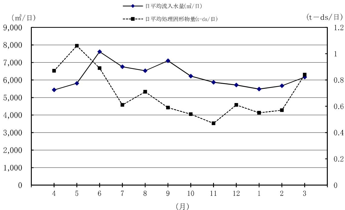
図6-7 令和5年度 流入水量・処理固形物量
