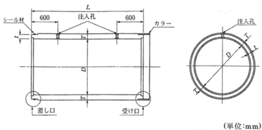
図 5-20 標準管の形状 (JSWAS A-2 P. 4)
