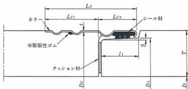
継手部詳細
