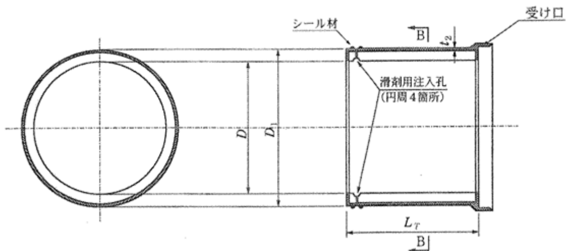
図 5－23 中押管 T の形状（JSWAS A-2 P. 7）
