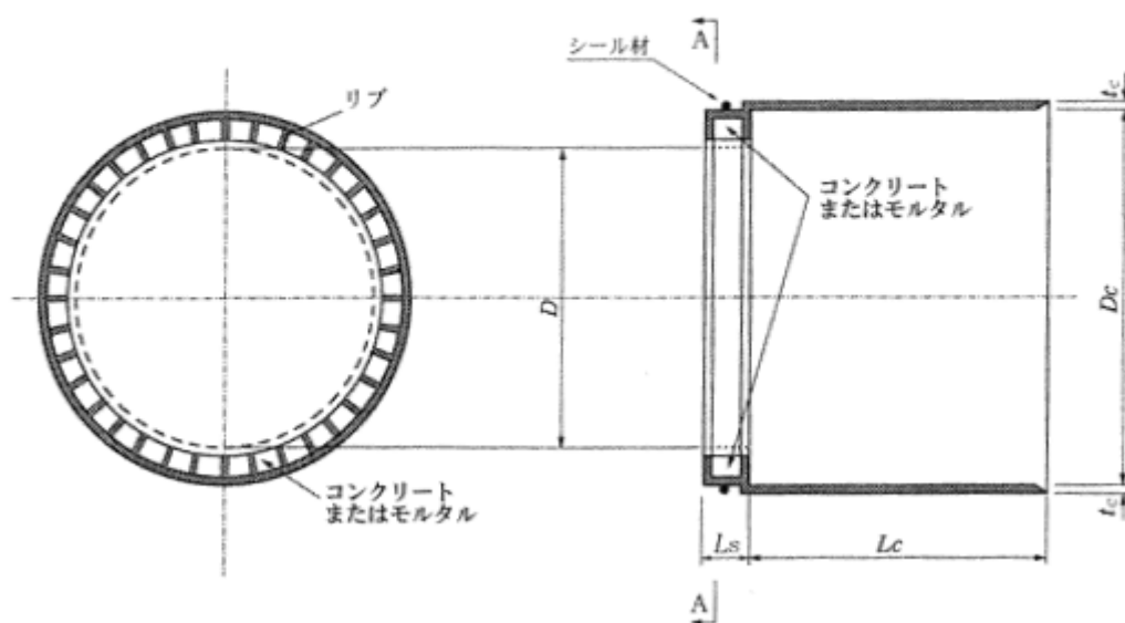
図 5 - 22 中押管 S の形状 (JSWAS A-2 P. 6)
