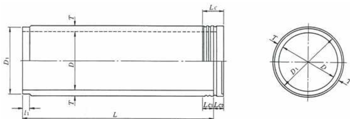
継手部詳細
