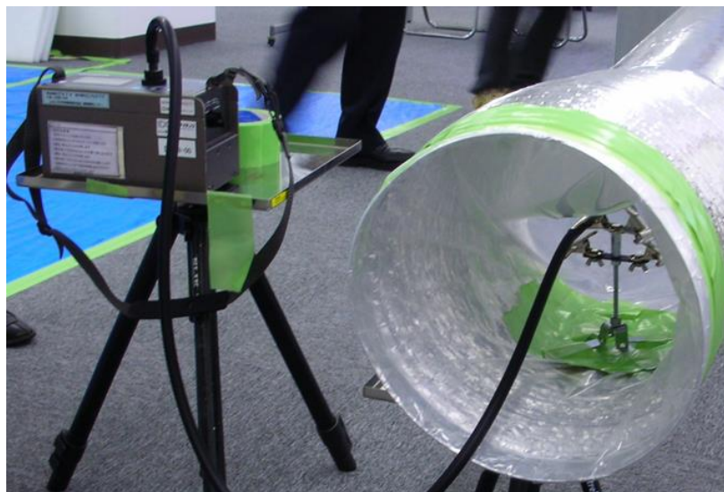
②集じん・排気装置が正常に稼働していることの確認方法の例 (デジタル粉じん計による確認)
