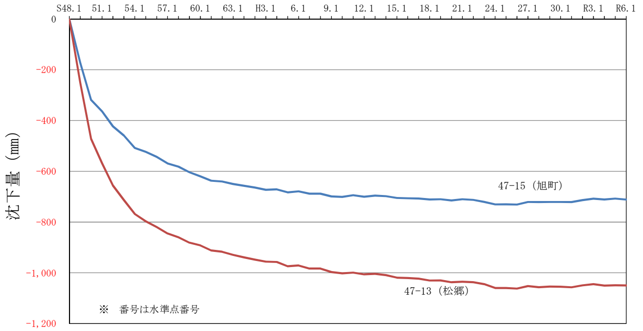
図 1 - 7 地盤沈下経年変化図 (所沢市) 測量基準日 (年. 月)
