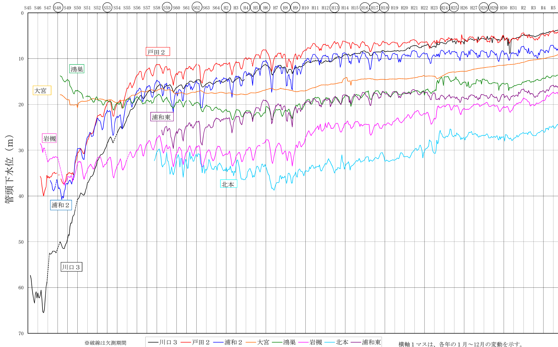
図 1-14 管頭下水位経年変化（中央部地域） (○印は渇水年)
