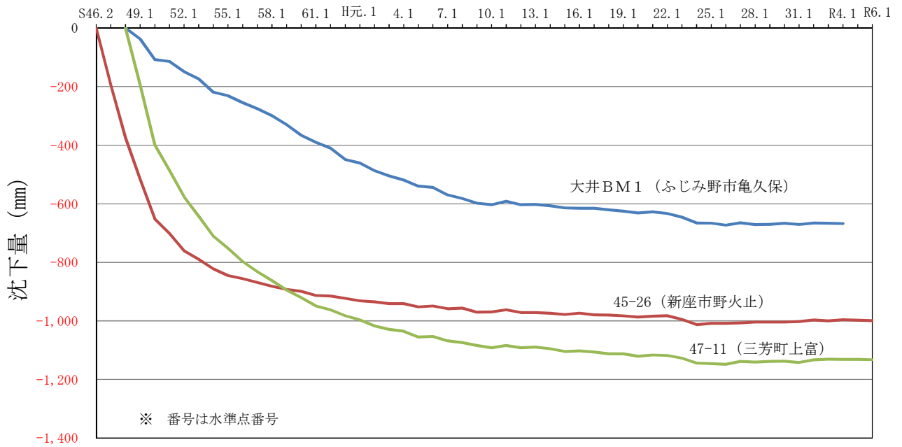
図 1 - 8 地盤沈下経年変化図 (ふじみ野市、新座市、三芳町) 測量基準日 (年. 月)
