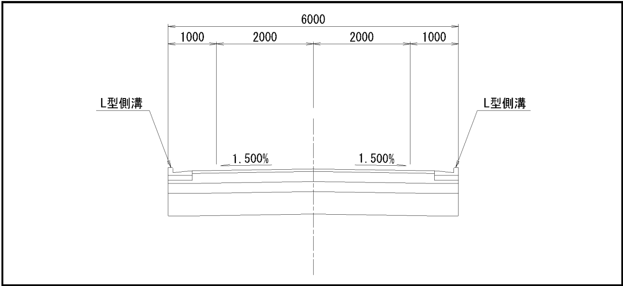
図 2.6-5(7) 道路の標準断面図 (区画道路 6m 幅員 6.0m)
