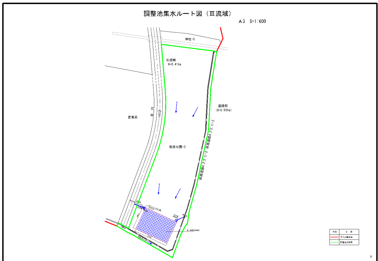
図 2.6-19 3号調整池集水ルート図
