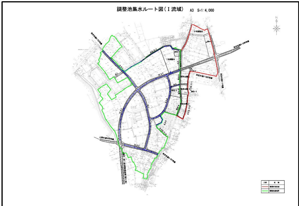
図 2.6-13 1号調整池集水ルート図
