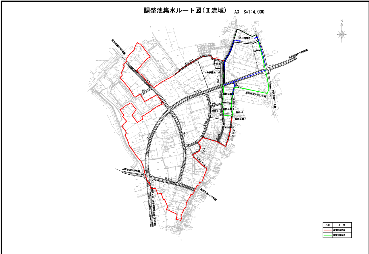
図 2.6-17 2号調整池集水ルート図
