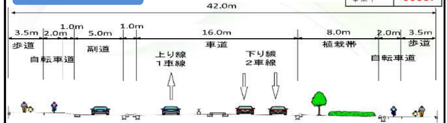
横断面(イメージ図)
