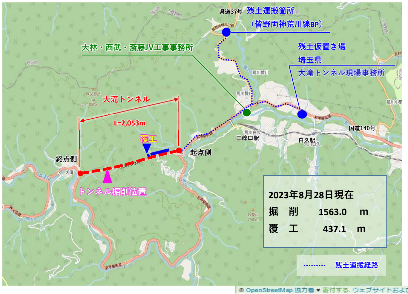
覆工 標準断面部が437m進みました。右写真は非常駐車帯（故障車等が退避する場所）取合い部を施工している所です。
