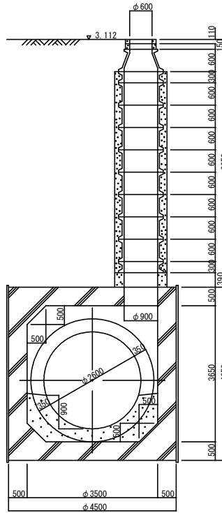
A-A断面図
