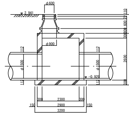
A-A断面図
