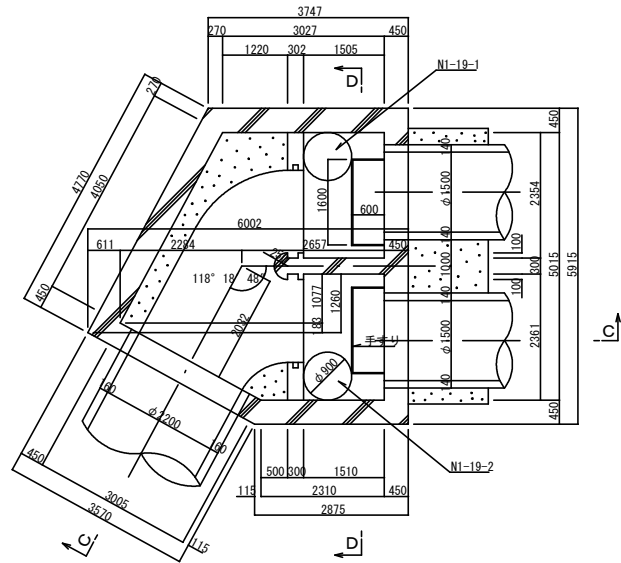
A-A平面図
