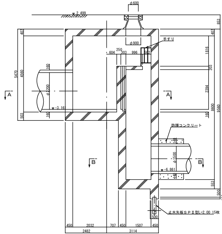
C-C断面図
