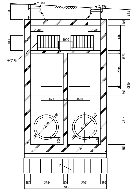
D-D断面図
