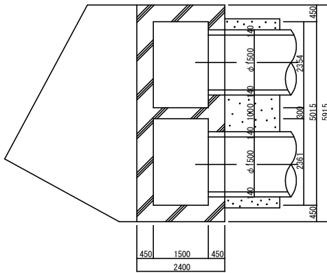
B-B平面図
