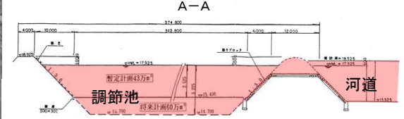
<調節池のイメージ>
