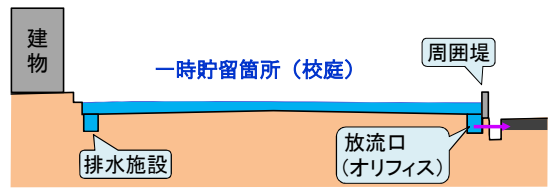
<校庭貯留（イメージ図）>
