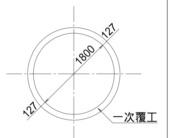
管渠断面図
