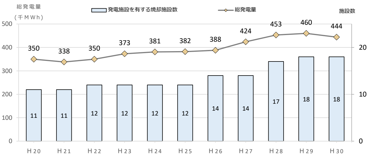
図 20 発電施設を有する焼却施設数及び総発電量の推移
