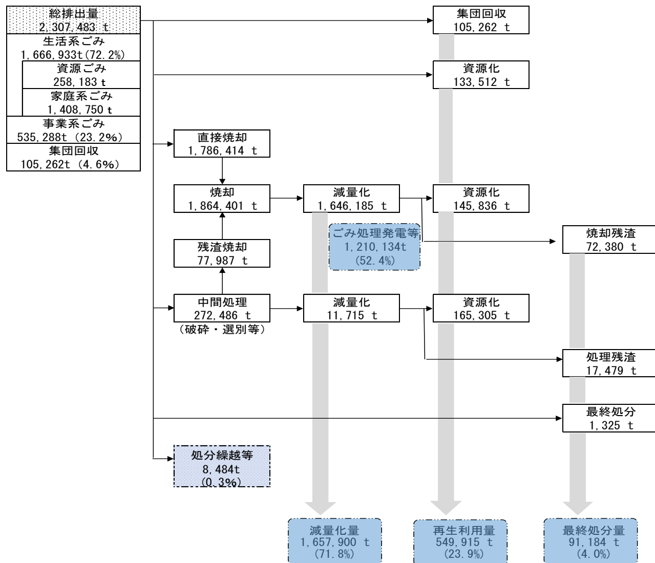
図3 ごみの処理・処分フロー（平成30年度）
