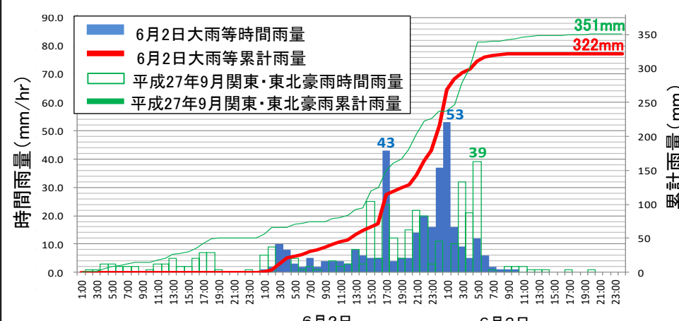
令和5年6月2日からの大雨及び台風第2号 2日間雨量と既往洪水の比較
