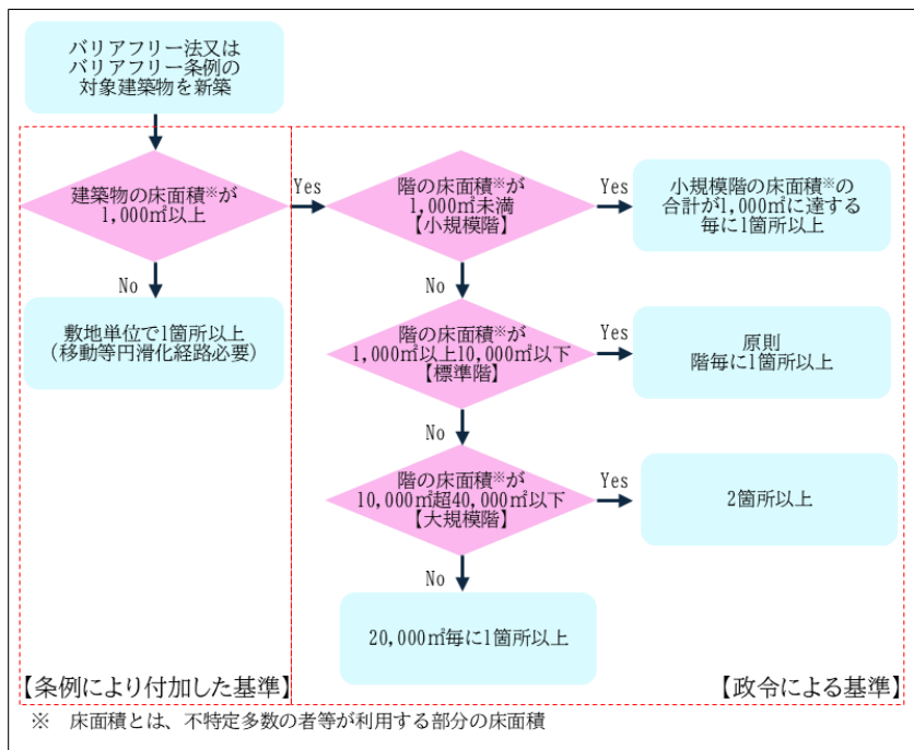
【別図2】車椅子使用者用便所の設置数算定フロー
