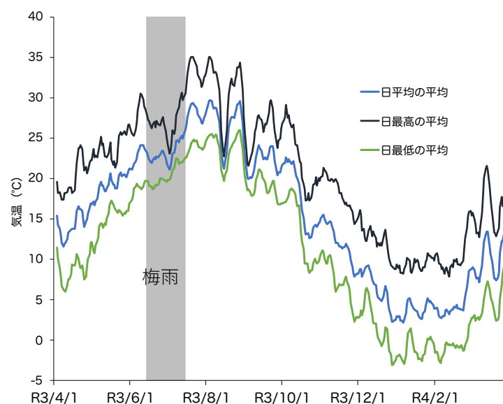
図6 令和3年度における本年度無欠測地点の日平均、日最高、日最低気温の平均値の推移(5日移動平均)
