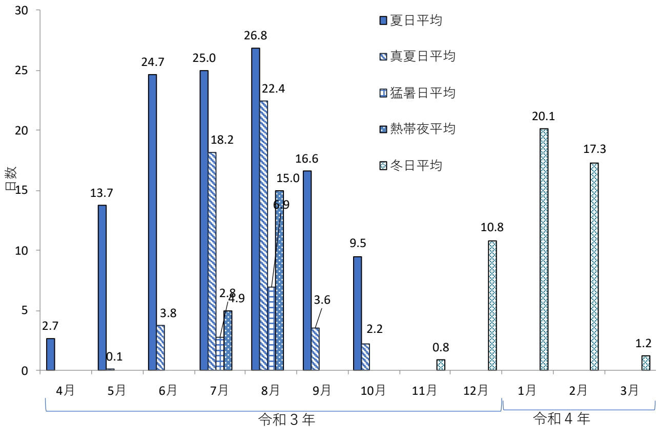
図7 令和3年度の長期観測点における夏日、真夏日、猛暑日、熱帯夜、冬日日数の月別平均値
