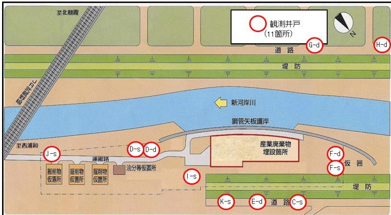
図 地下水の試料採取位置
