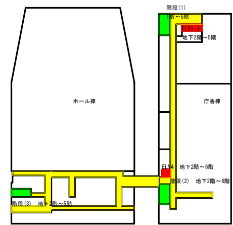
5階平面図
