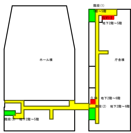
4階平面図
