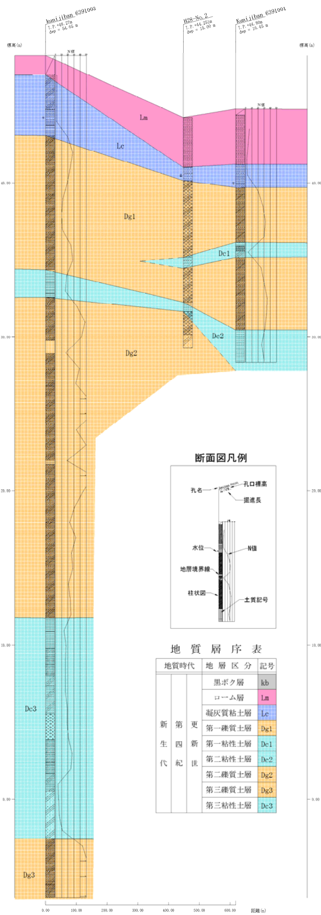
図 2-20 地質想定断面図 ④-④' 断面
