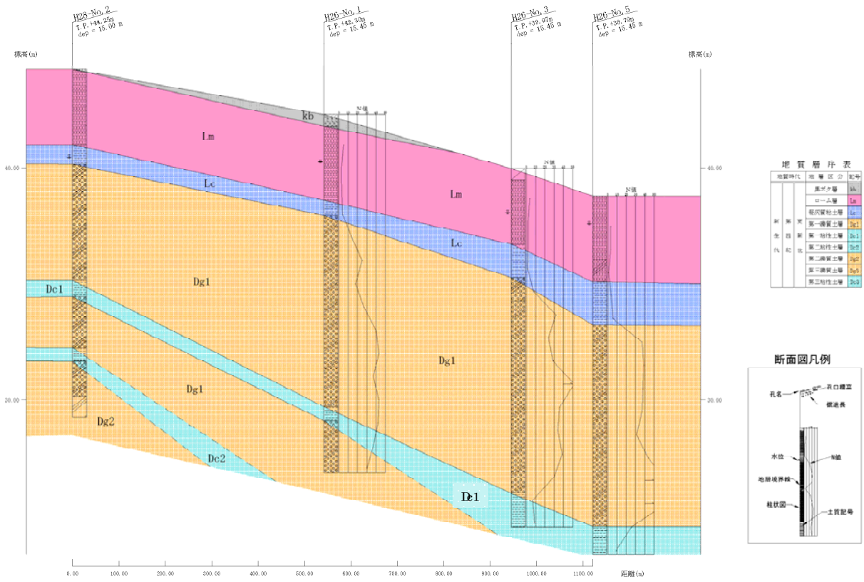
图 2-17 地質想定断面图 ①-①' 断面
