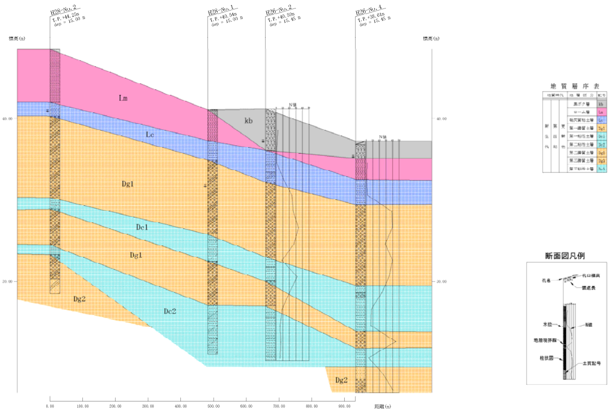
图 2-18 地質想定断面图 ②-②' 断面
