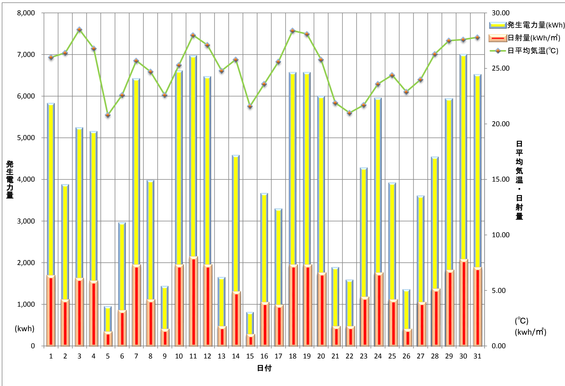
行田浄水場 太陽光発電量 (2016.7)
