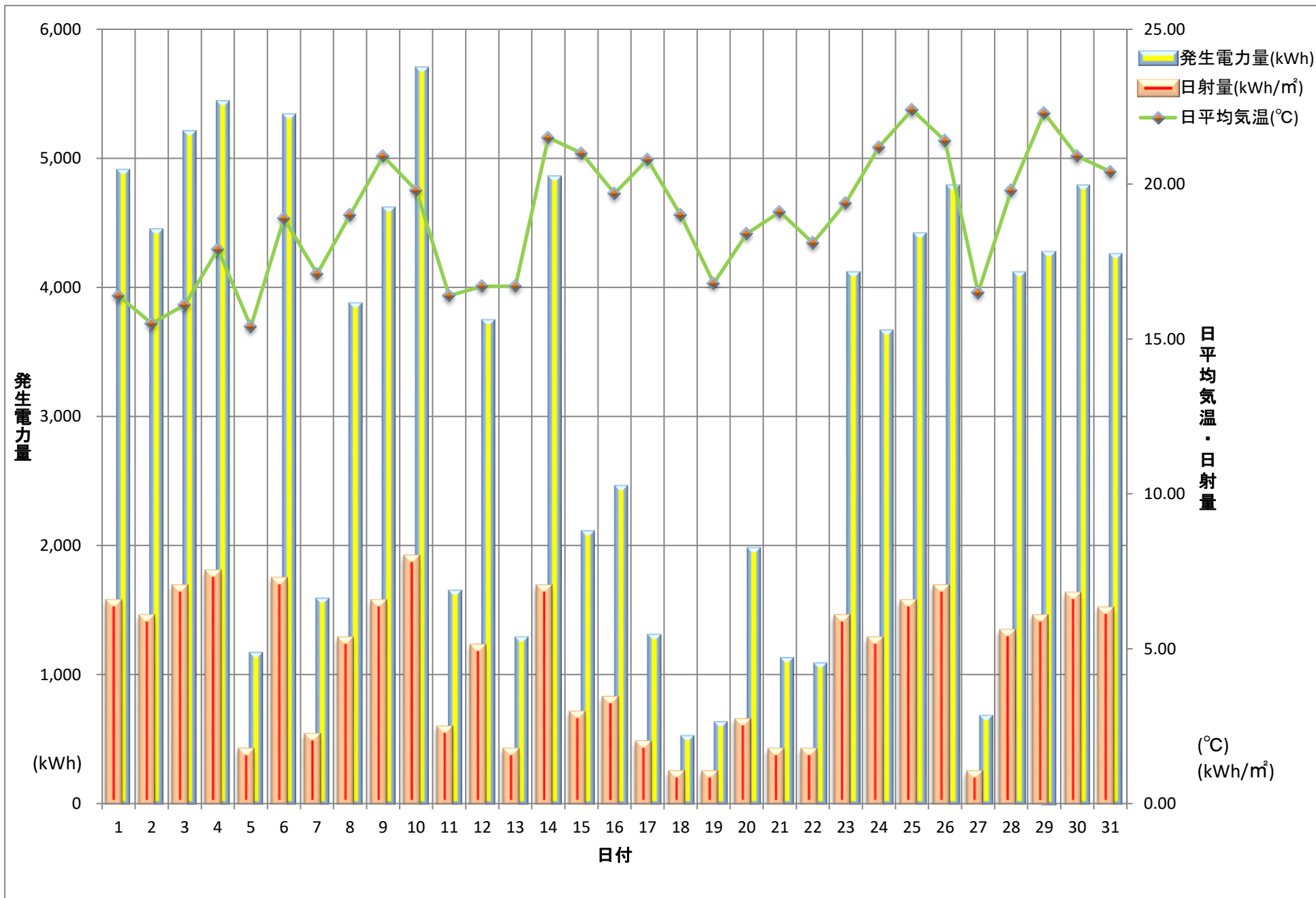
行田浄水場 太陽光発電量 (2021.5)
