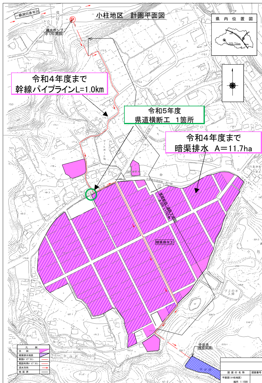
小柱地区 計画平面図
