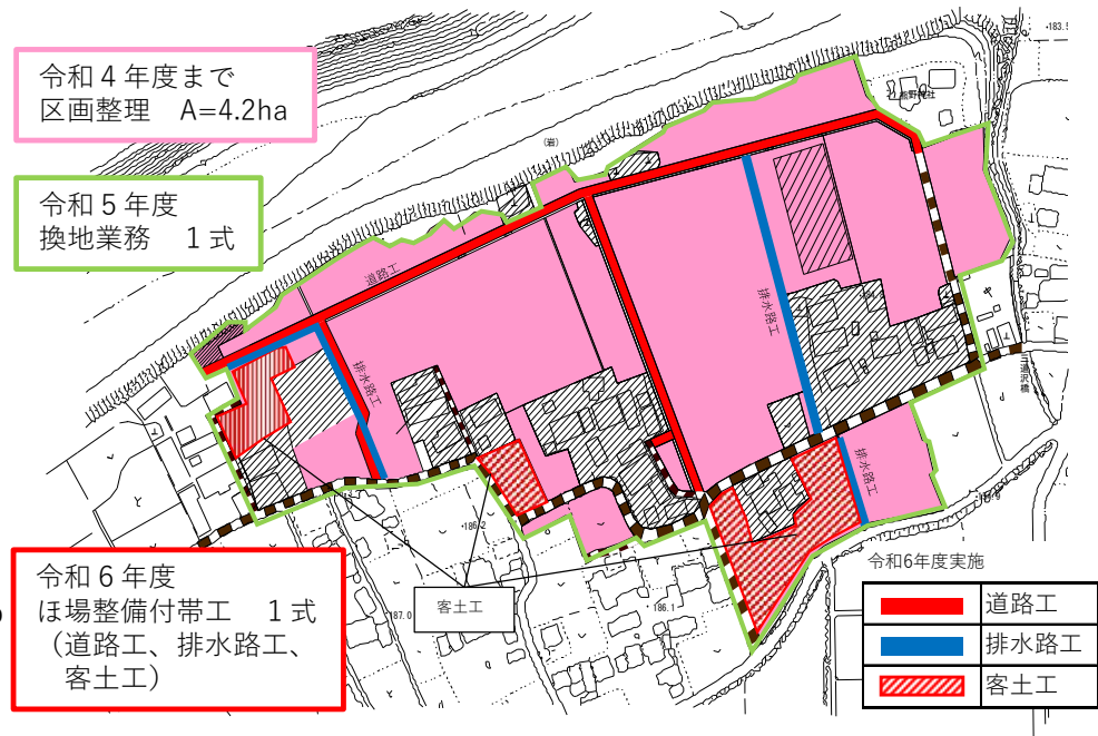
中太田地区 計画平面図
