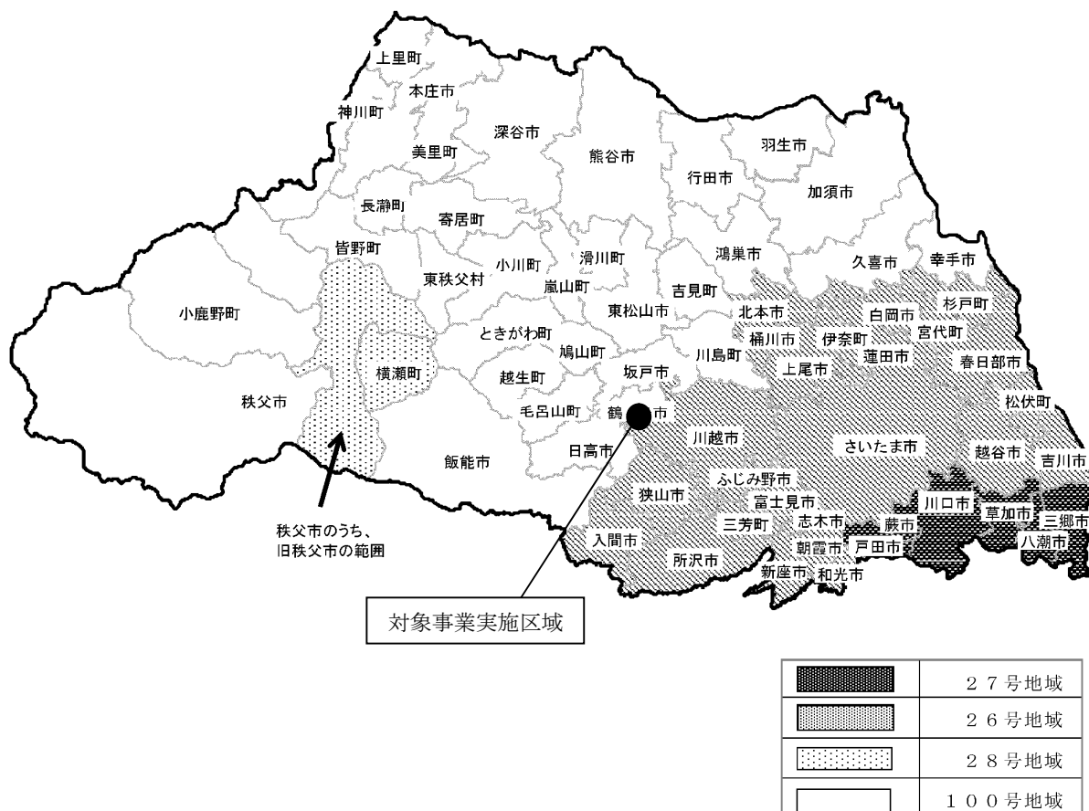
図 3-20 硫黄酸化物に係る K 値規制図
